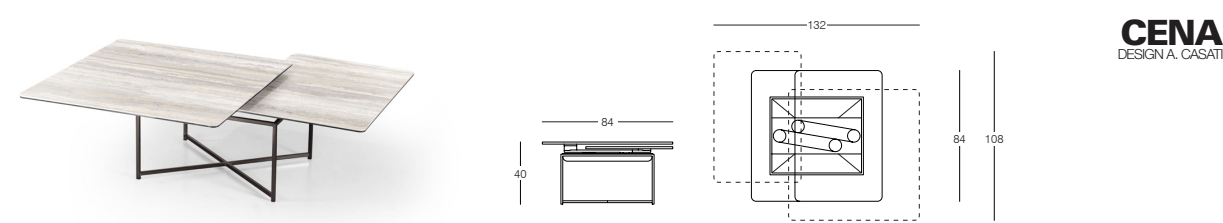
CENA. AUSZIEHBARER COUCHTISCH MIT KERAMIKPLATTEN. BASIS AUS LACKIERTEM ODER GALVANISIERTEM STAHL. AUSGESTATTET MIT EINEM INNOVATIVEN MECHANISMUS, DIE ERMÖGLICHT DIE 2 UNTERE REGALE ZU ÖFFNEN.
