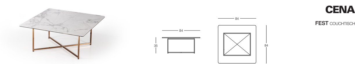
CENA. FEST COUCHTISCH MIT KERAMIKPLATTE. BASIS AUS LACKIERTEM ODER GALVANISIERTEM STAHL.
