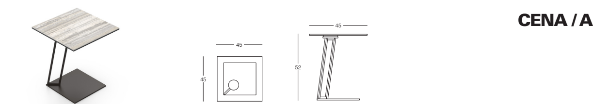
CENA / A. BEISTELLTISCH MIT KERAMIKPLATTE . GESTELL AUS LACKIERTEM STAHL.
