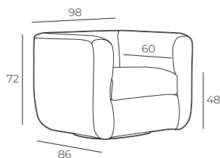
Stuhl mit swivel mechanismus STORMY WITH SWIVEL
